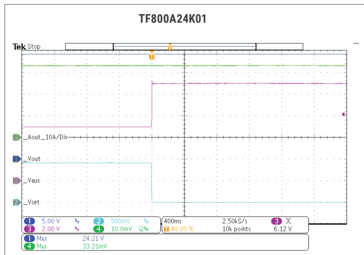
Fig. 59: (Vset Hi-Lo)(Vaux 9V-5V) 230VAC.
