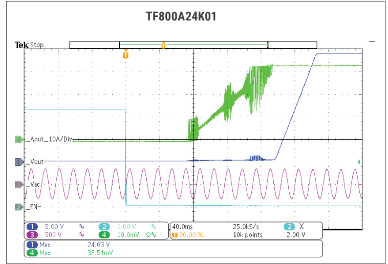
Fig. 53: INHIBIT (EN-)Lo Vout On 230VAC.
